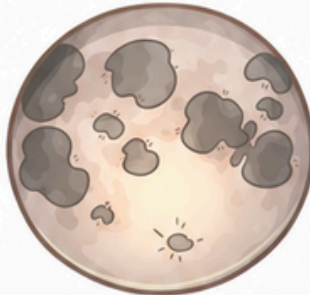
Moon
