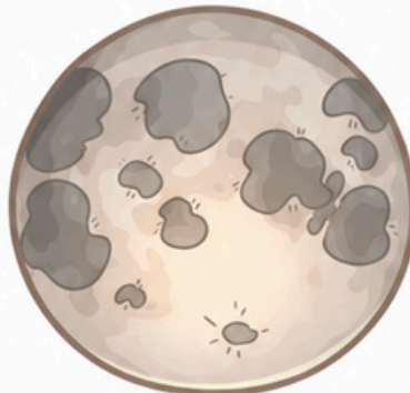
Moon
