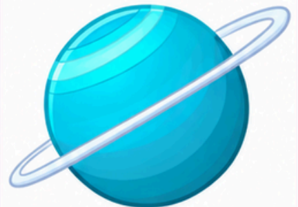
Uranus
