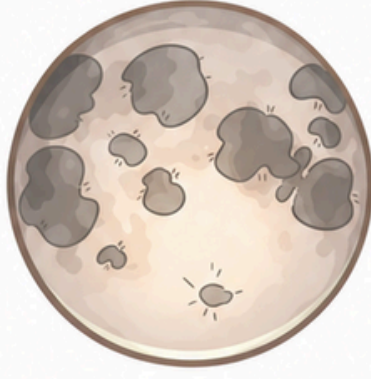
Moon
