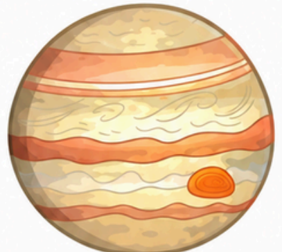
Jupiter
