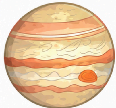
Jupiter
