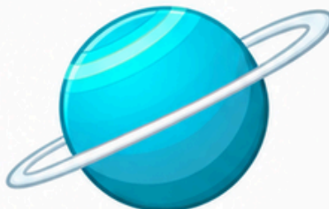
Uranus
